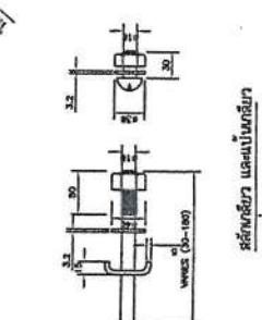
รูปตัดขวางแบบแปลน มาตราส่วน 1 : 3
